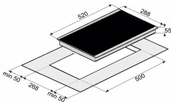
Einbauskeizze
