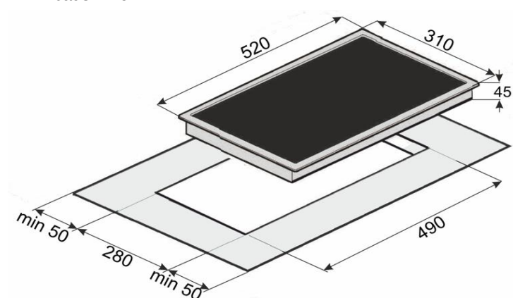
Einbauskizze
